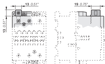
LK75-L, LK110
