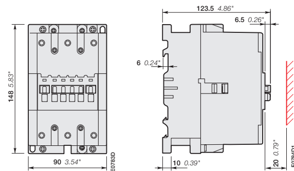
AF95, AF110
