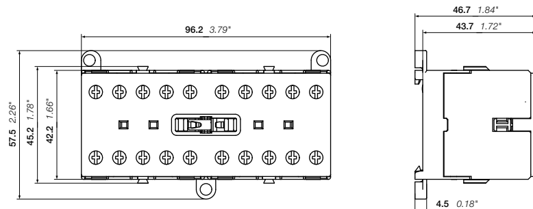
VB6, VB7
