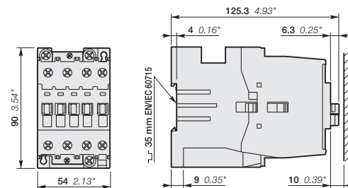
AL40
