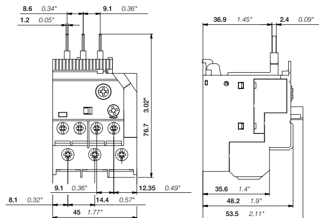
T16
