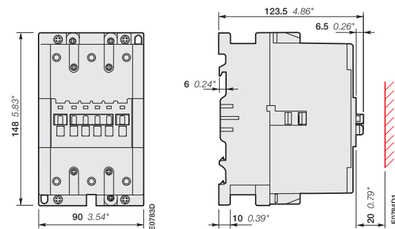
A95, A110
