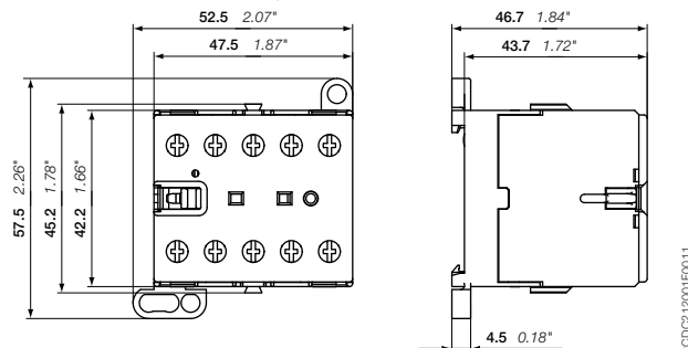
TBC7
