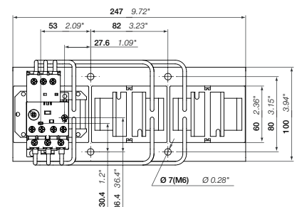
E800DU
