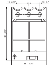
DB80
