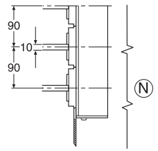
E1 View A
