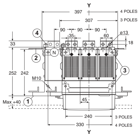
E1/E2 View A
