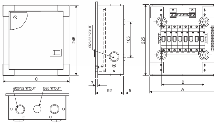
IP43 Double Door – Metal Door
