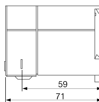
DIN RAIL TYPE
