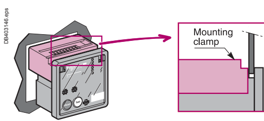
Front-panel mount.
