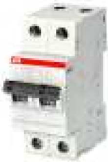
SB202 M C 16
