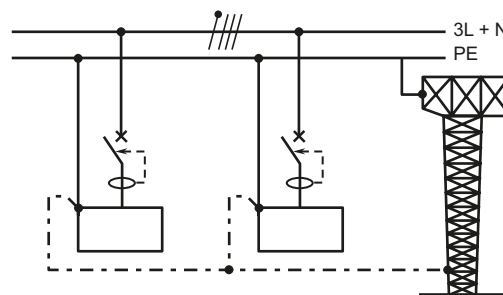
Fig. F31 Improved equipotential bonding
