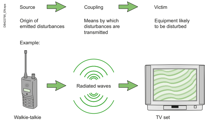
Fig. R29 EM interference phenomenon
