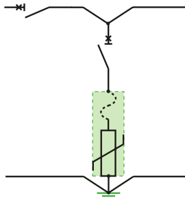
Fig. J34 SCPD «in parallel»
