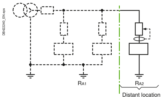
Fig. F16 Separate earth electrode
