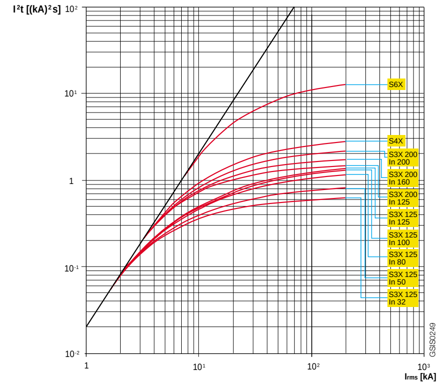
SACE Isomax S3X 125 – S3X 200 – S4X – S6X – 400-440V
