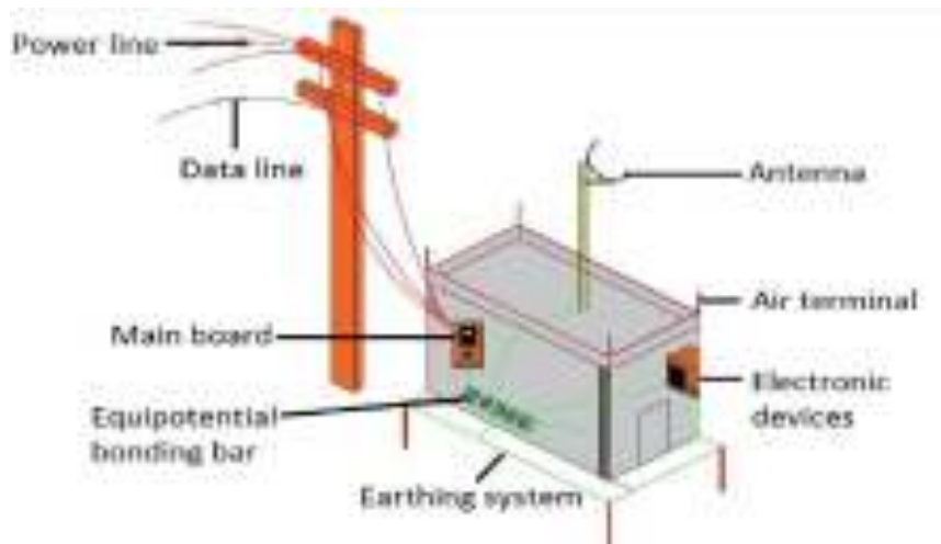
Figure 33. Equipotential bonding
