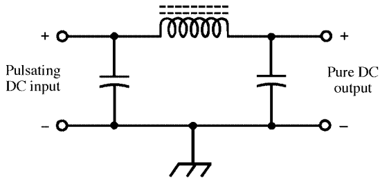
rectifier filter
