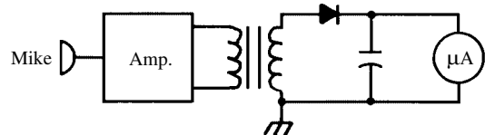
noise meter
