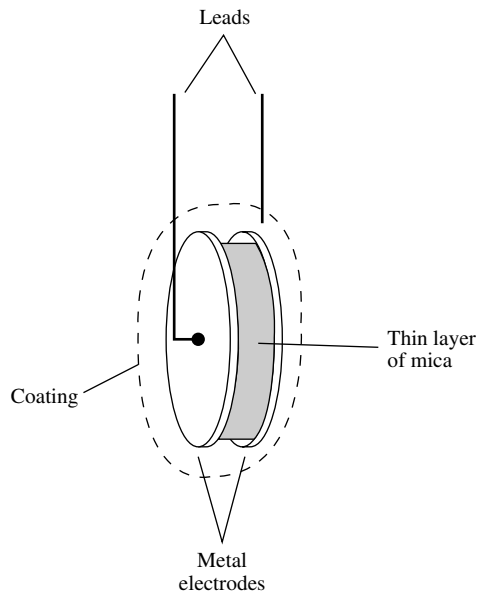
mica capacitor
