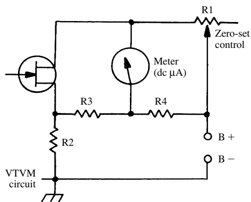
zero set, 2
