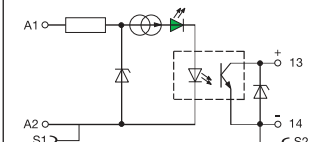
OB...IC 0100 - 5-12 V DC 115-230 V AC/DC
