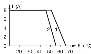
RB 121 A 110-220 VAC/DC 1 : 110 V AC/DC block 2 : 220 V AC block
