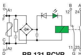
RB 131 BCVR
