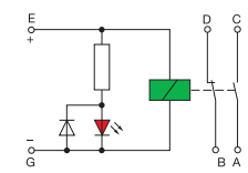
RB 131
