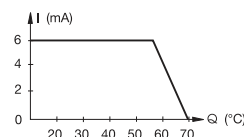
OBC 0100 S
