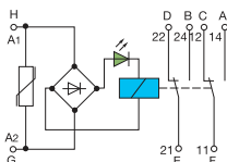
RB 122 A
