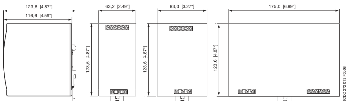
CP-E 12/10.0, CP-E 24/5.0
