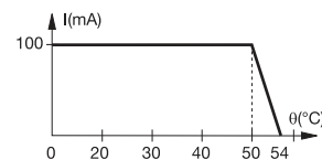
D 2,5/5-OB0C-0100 48 V DC
