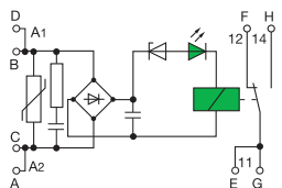
RB 121 BCVR
