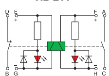
RB 310
