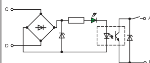
OBC 0100 S
