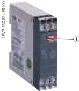
CM-PFE
