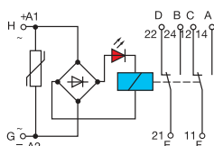
RB 122 AV
