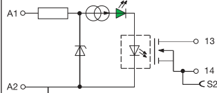
OB...OC 1000 - 5-12 V DC
