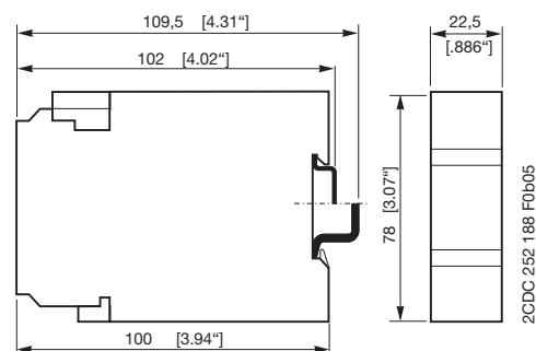
CP-RUD
