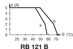
RB 121 B
