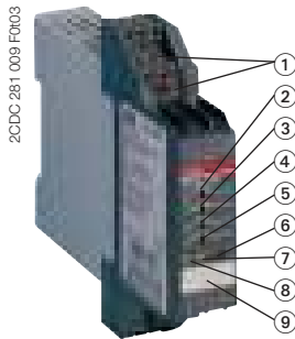
CC-U/TCR
