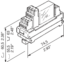
RM 122 B - 115/220 V AC
