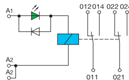
RM 122 B - 115/220 V AC
