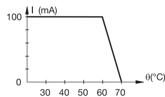
OBC 0100
