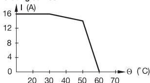
RM 121 24 V DC
