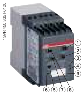
CM-LWN
