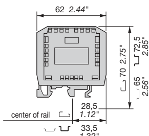
RB 131
