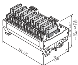
RM 821...
