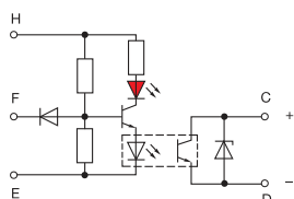
EB ODC
