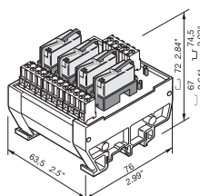
RM 421...
