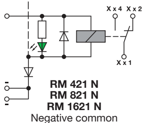
RM 1621...
