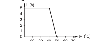
RB 121 CV RB 121 BCVR
