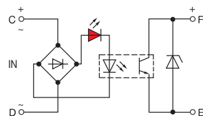
EBO1...
