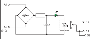
OB...OC 1500 - 24 V AC/DC OB...OC 1000 - 24 V DC 48-60-115-230 V AC/DC
