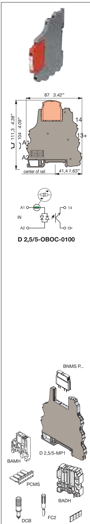
D 2,5/5-OB0C-0100 5 V DC / 24 V DC
