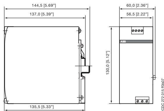
CP-A RU
