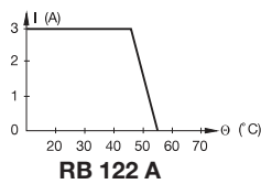
RB 122 A
