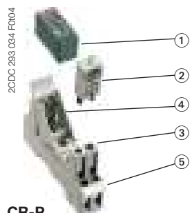
CR-P
