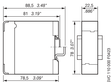
CM-E 22.5 mm
