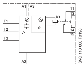
C510
