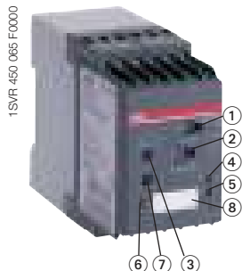
CM-IWN-DC
