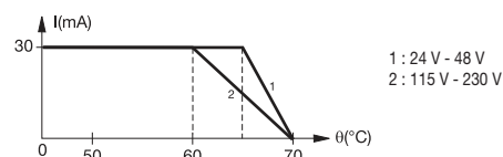
D 2,5/5-OBIA-0030
